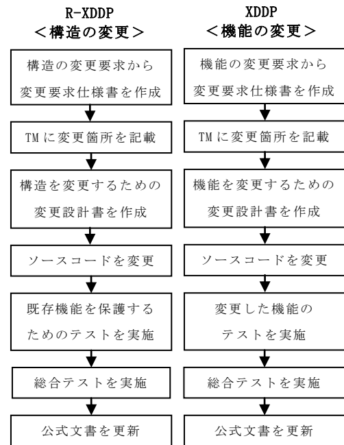
図 3 構造の変更と機能の変更プロセス
