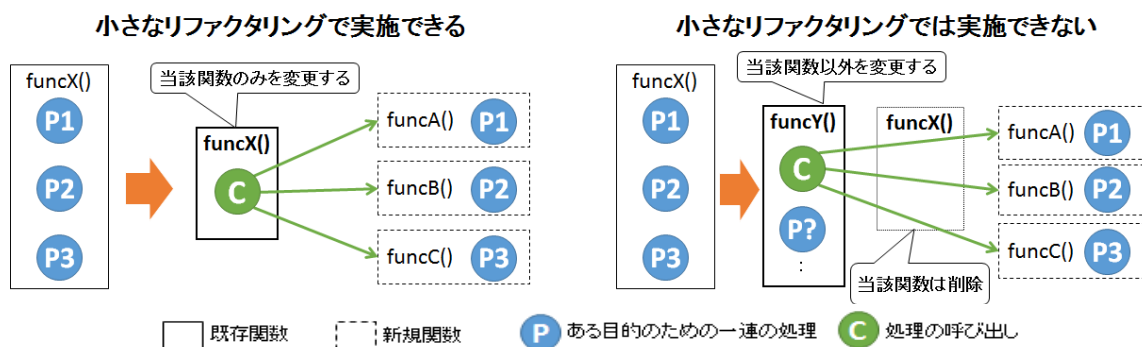
図2 小さなリファクタリングで実施できるパターンと実施できないパターン
