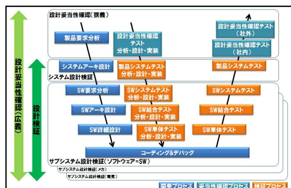
図 1-1.設計妥当性確認と設計検証の構造
