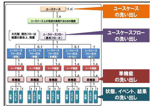
図 2-1. ユースケースの体系図
